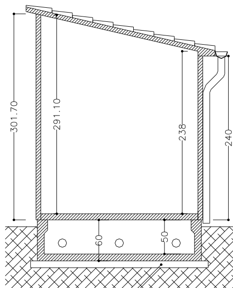
SEZIONE
