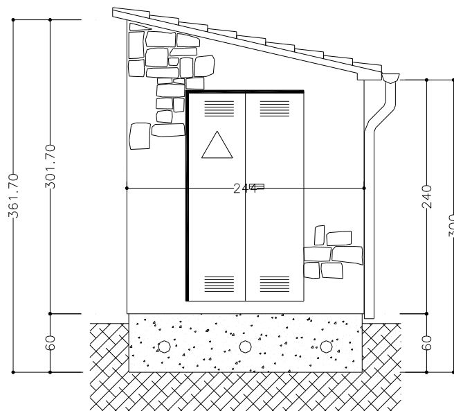
LATO SINISTRO
