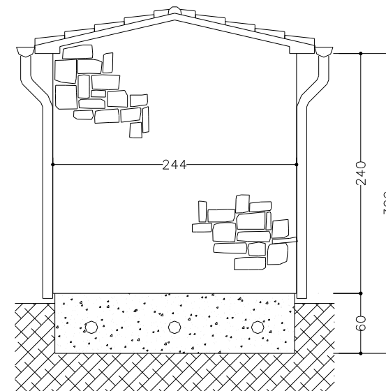
LATO DESTRO
