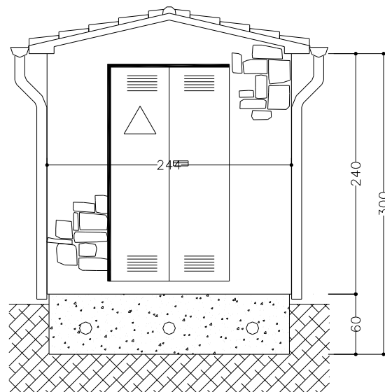
LATO SINISTRO
