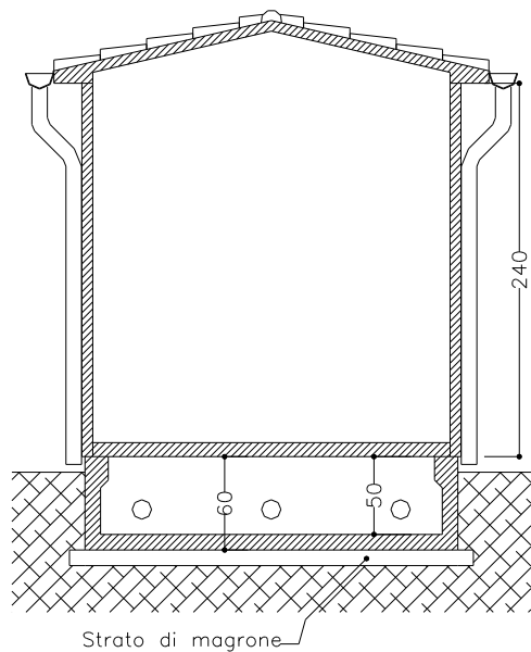
SEZIONE
